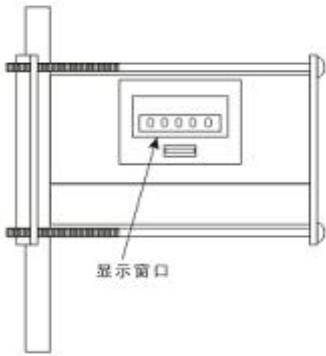
图2：安装侧面
