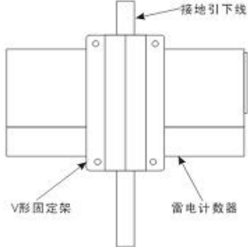
图3：安装背面
